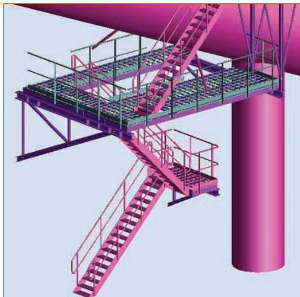
New platform for access to flue gas duct; Vestforbrændingen I/S
